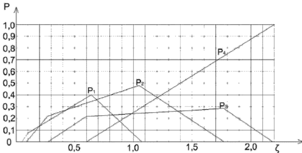
Рисунок 4.1 - Вероятности различной степени разрушения здания (сооружения) и повреждения технологического оборудования в зависимости от величины обобщенного показателя устойчивости, \xi_{об}(\xi_{то})
