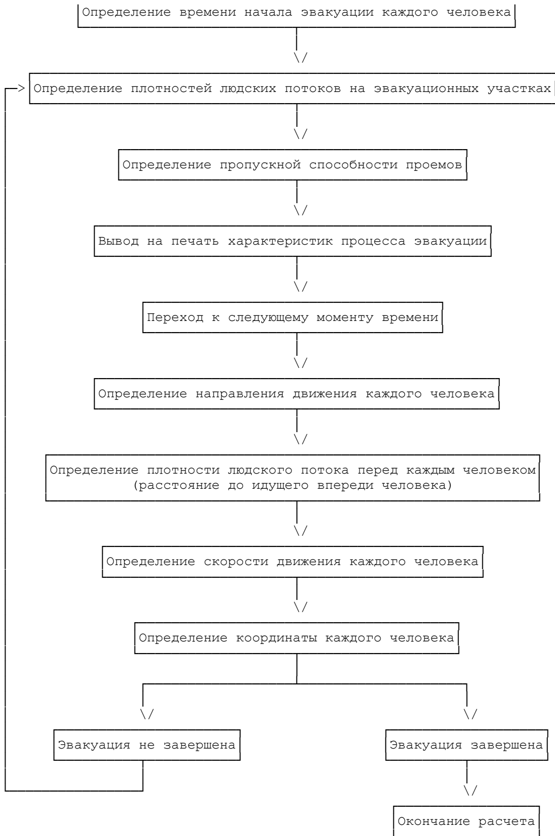
Рис. ПЗ.2. Блок-схема определения расчетного времени эвакуации людей из здания
