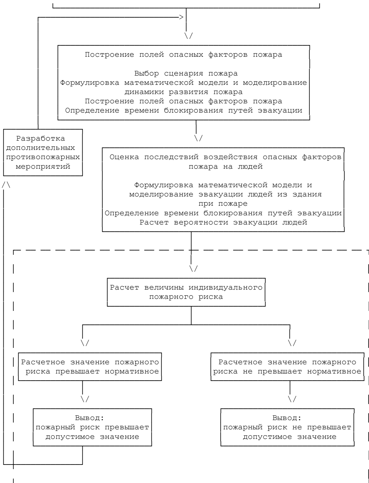
Рис. 1. Порядок проведения расчета индивидуального пожарного риска
