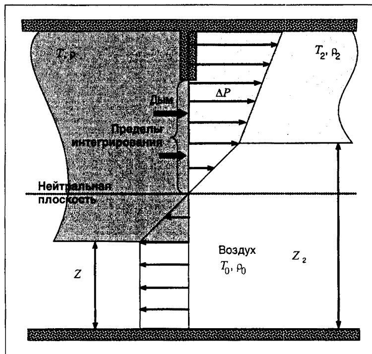
Рис. Пб.1. Массопотоки через проем
