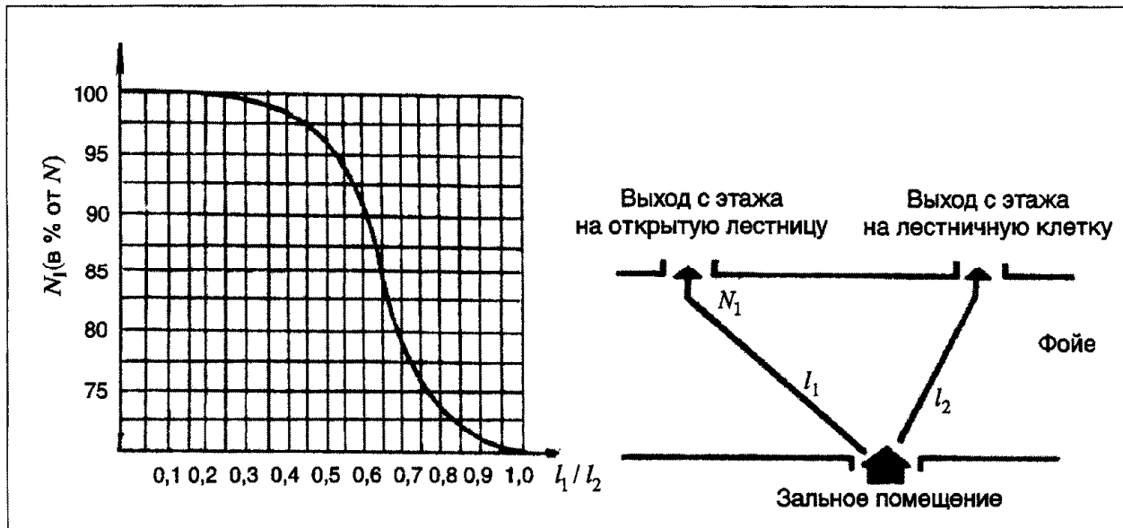
Рис. П5.5, б. Число зрителей, эвакуирующихся по открытой лестнице: N - общее количество эвакуирующихся; N_1 - число эвакуирующихся по открытой лестнице; l_1 - длина пути до открытой лестницы; l_2 - длина пути до выхода на лестничную клетку
